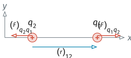
Figura 3: Sistema de dos cargas eléctricas. Podemos ver sus vectores de posición y la fuerza eléctrica resultante. Elaboración propia.
