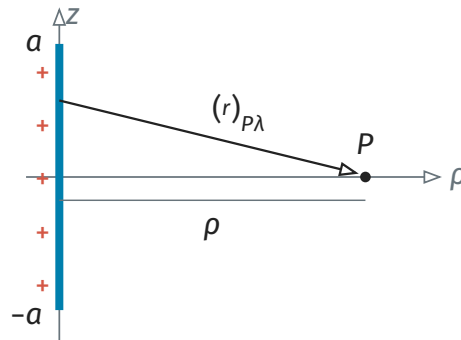
Figura 5: Campo de una carga. Elaboración propia.
